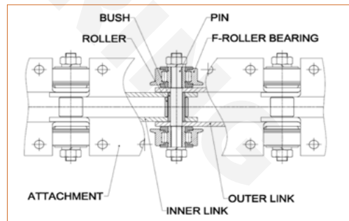
F-롤러 베어링
