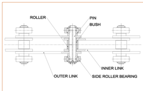
사이드 롤러 베어링
