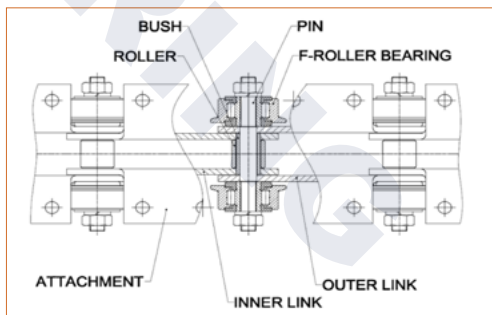
F-롤러 베어링
