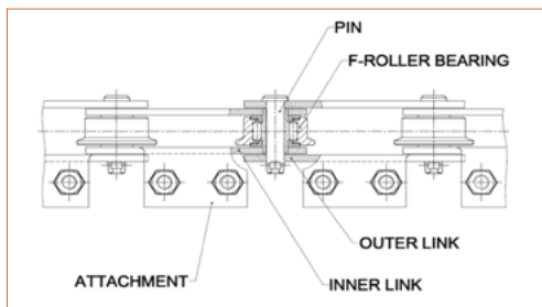
F-롤러 베어링
